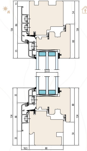
SYSTEM NATURO 80 ALU GEMINI CLASSIC Innen- und Außenfensterbankfräsung
