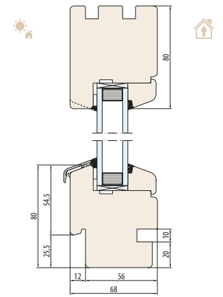
SYSTEM NATURO 68-Fix Innen- und AußenFensterbankfräsung
