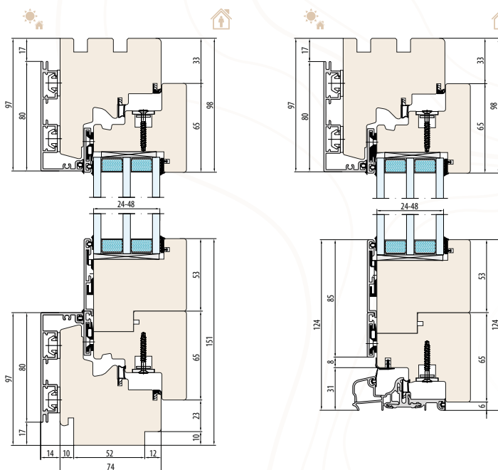
SYSTEM ESPERIA LIFE 74 ALU Einfügelige Balkontüren mit hoher Schwelle
