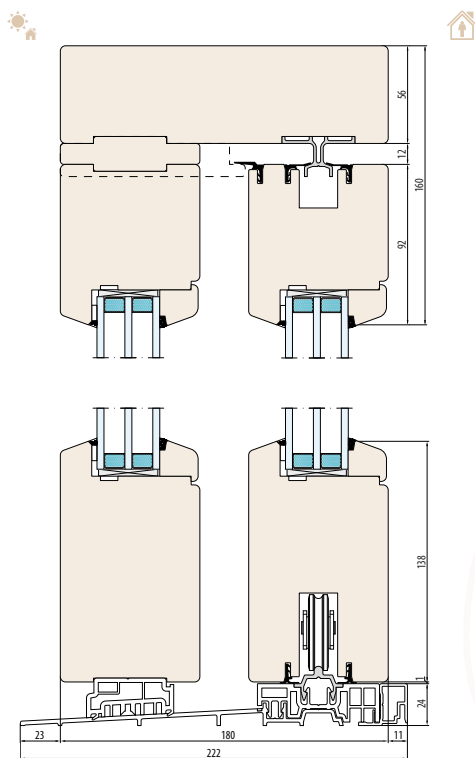
SYSTEM NATURO 80 HST (Allgemeine Maße) - Schwelle 24 mm - Schema "A"
