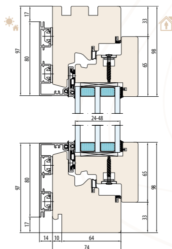
SYSTEM ESPERIA LIFE 74 ALU Äußere Fensterbankfräsung
