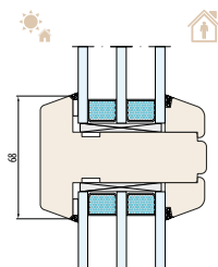
SYSTEM NATURO 92 Konstruktionssprosse 68 mm
