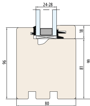
SYSTEM ESPERIA LIFE 80-Fix Ohne Fensterbankfräsung
