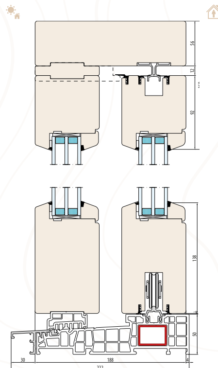
SYSTEM NATURO 80 HST (Allgemeine Maße) - Schwelle 50 mm - Schema "A"
